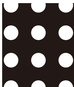
75 8.0φ × 15.0P 開孔率 22.3%
