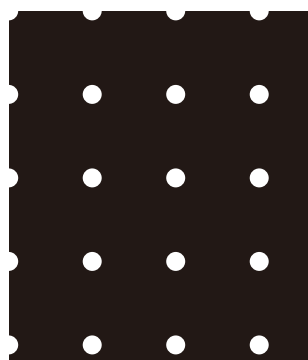
63 2.5φ × 11.0P 開孔率 4.1%
