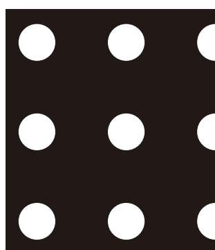
73 7.0φ × 17.0P 開孔率 13.3%
