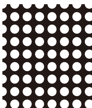
66 4.0φ × 5.5P 開孔率 41.5%
