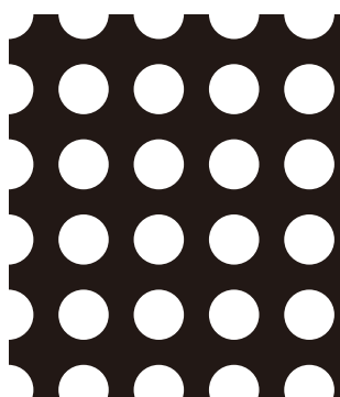
70 6.0φ × 9.0P 開孔率 34.9%
