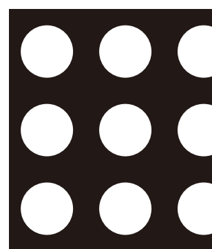
76 10.0φ × 15.0P 開孔率 34.9%
