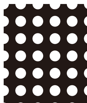
68 5.0φ × 8.0P 開孔率 30.7%
