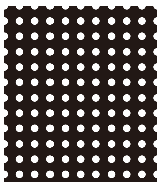
61 2.0φ × 4.0P 開孔率 19.6%
