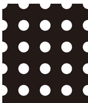
69 5.0φ × 10.0P 開孔率 19.6%
